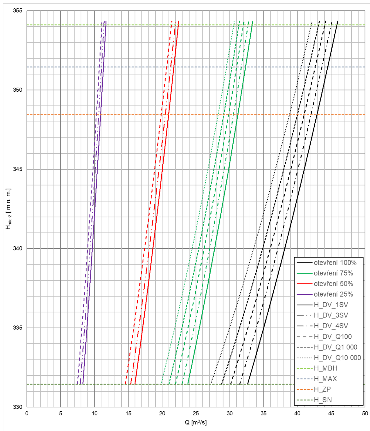
Obr. 1 – Měrná křivka průtoků spodní výpustí pro 100%, 75%, 50% a 25 % otevření SG uzávěru a pro různé dolní vody
