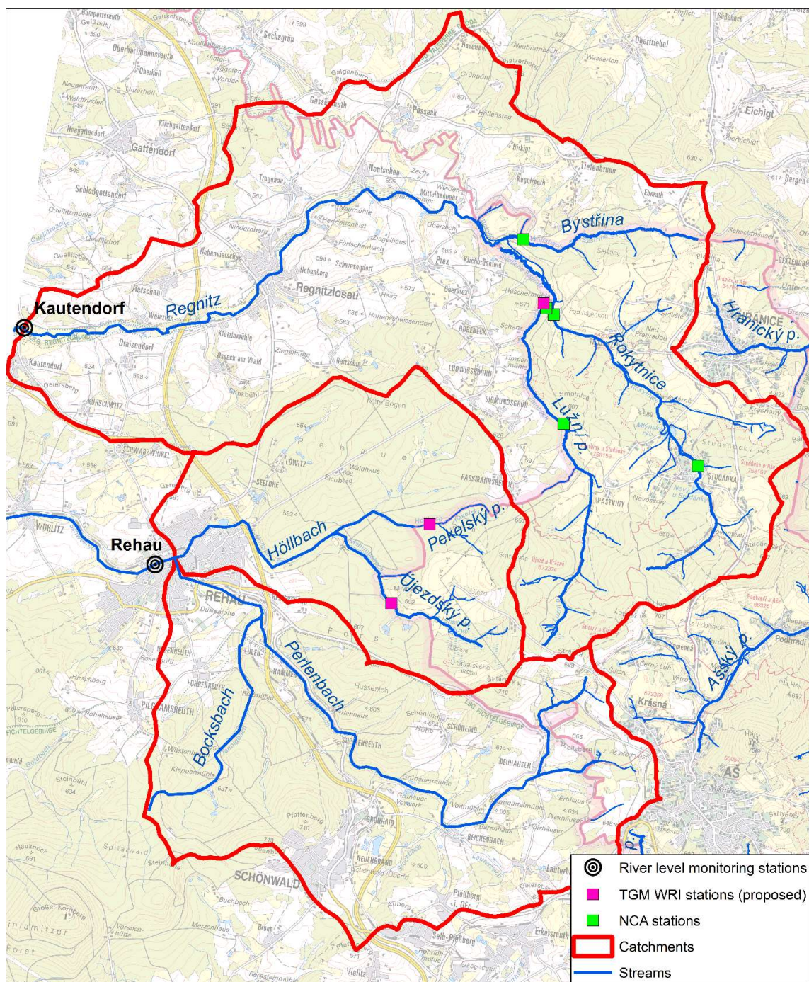
Obrázek 20. Vodoměrné stanice na německém území (Kautendorf a Rehau) a stanice VÚV TGM (TGM WRI Stations) a AOPK ČR (NCA Stations)
