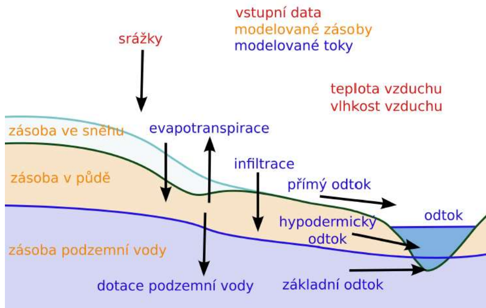
Obrázek 25. Schéma hydrologického modelu Bilan
