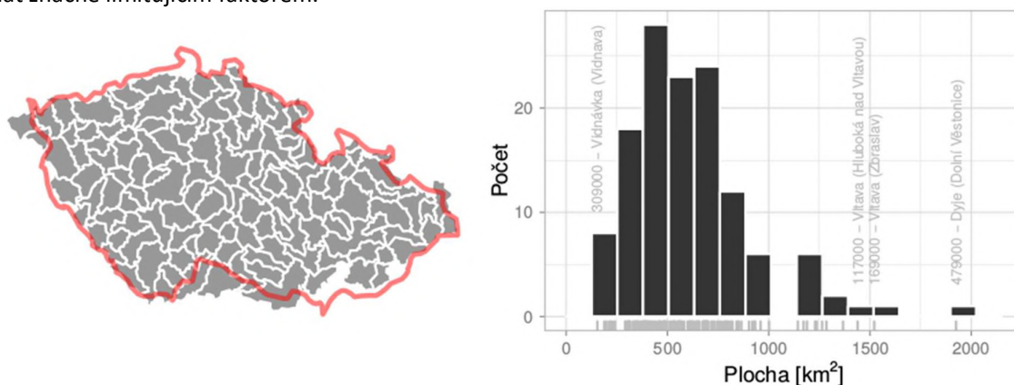
Obrázek 34. Vybraná sada povodí (vlevo) a jejich rozloha (vpravo).
