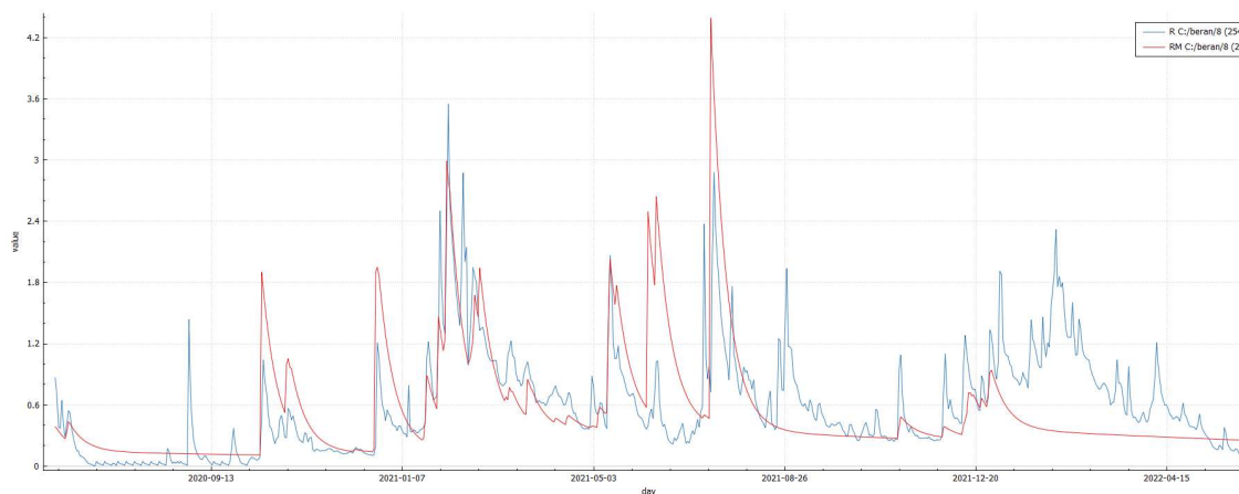
Obrázek 29 Pozorovaný (modře) a modelovaný (červeně) odtok z povodí Rokytnice (11. 6. 2020 – 31. 5. 2022)
