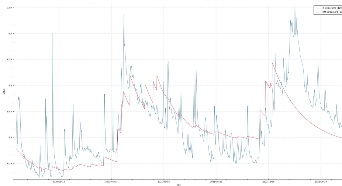
Obrázek 26. Pozorovaný (modře) a modelovaný (červeně) odtok z povodí Újezdského potoka (11. 6. 2020 – 31. 5. 2022)
