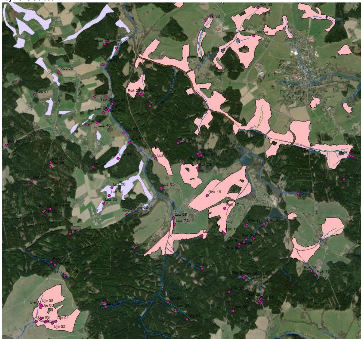
Obrázek 6. Překryv pramenišť, zmapovaných v letech 2020 – 22 v zájmovém území s mapou ploch, odvozených během systematických meliorací ve 2. polovině 20. století (zdroj VÚMOP a WWA Hof)
