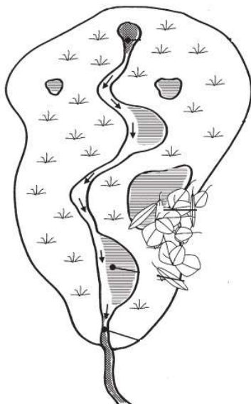
Obrázek 4. Schéma helokrenního prameniště (pramenného mokřadu)
