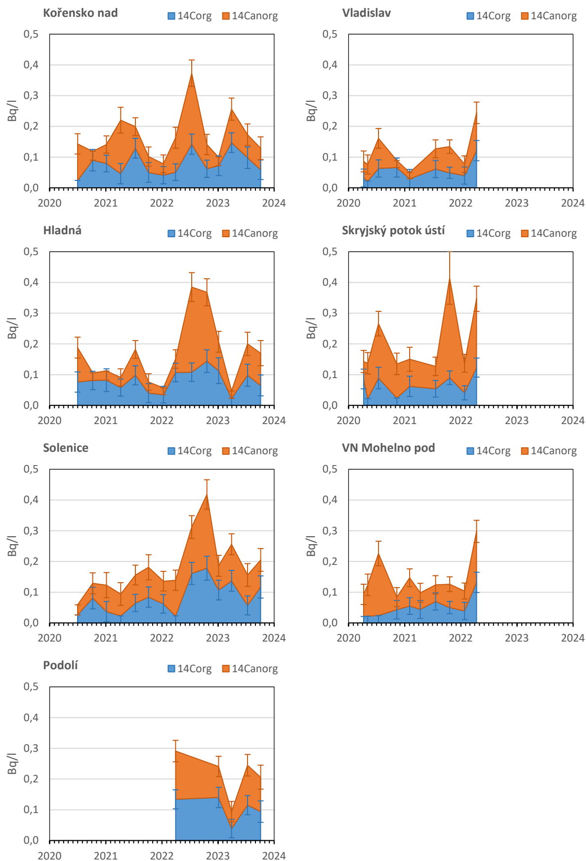
Obr. 3. Časový průběh naměřených hodnot jednotlivých forem ^{14}\text{C} je pro jednotlivé sledované profily
